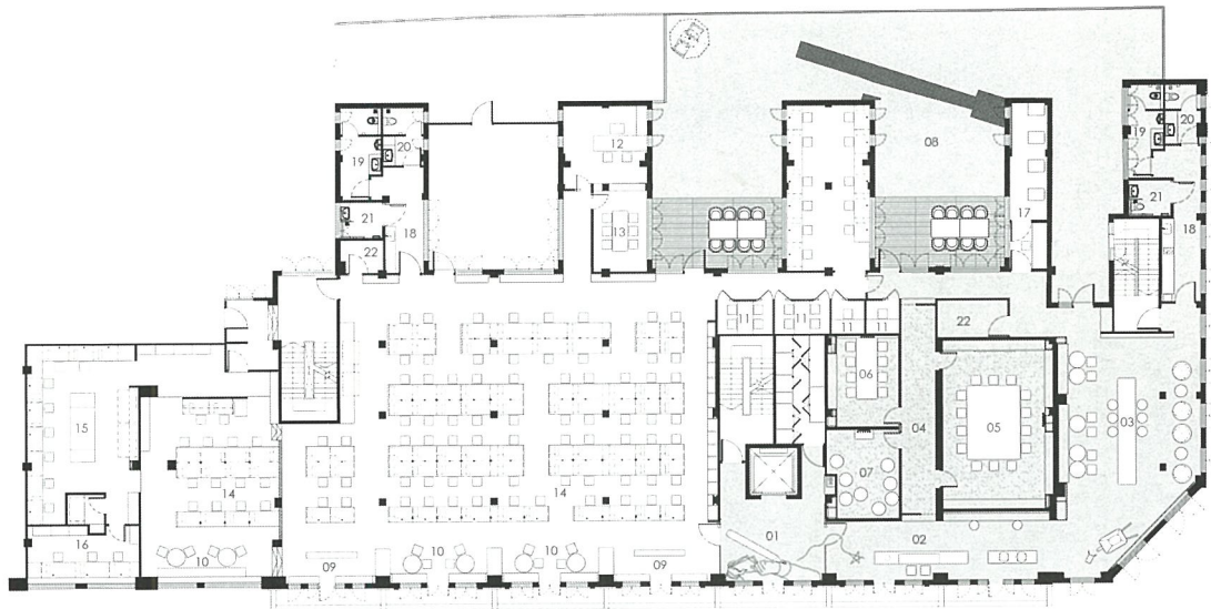
平面布置图
